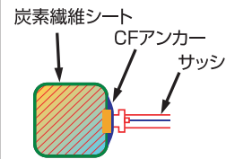
サッシを付けたままの補強
